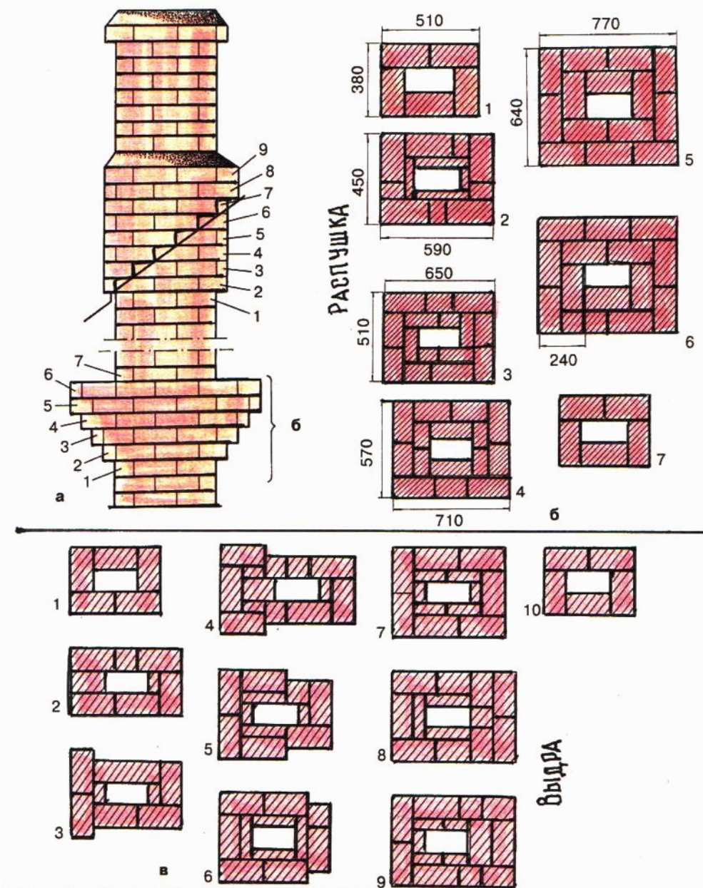
Рис. Кладка распушки и выдры с дымовым каналом 140x270 мм: а — общий вид трубы; б — порядовки распушки; в — порядовка выдры с дымовым каналом 140x270 мм
